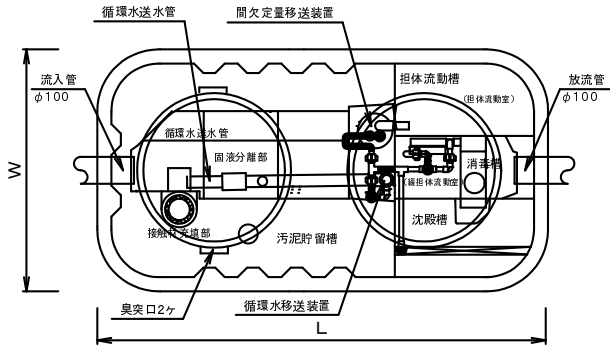
平面図
