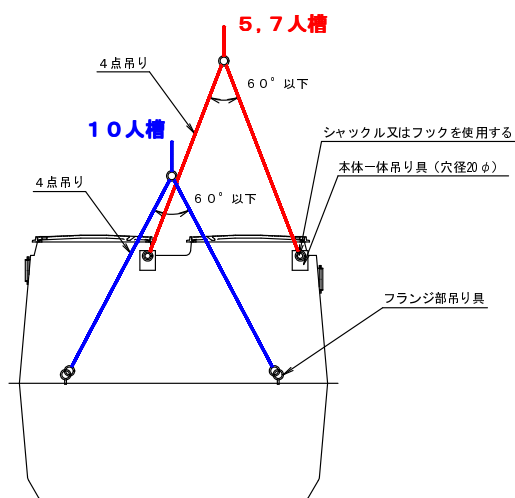
ワイヤーロープの掛け方
