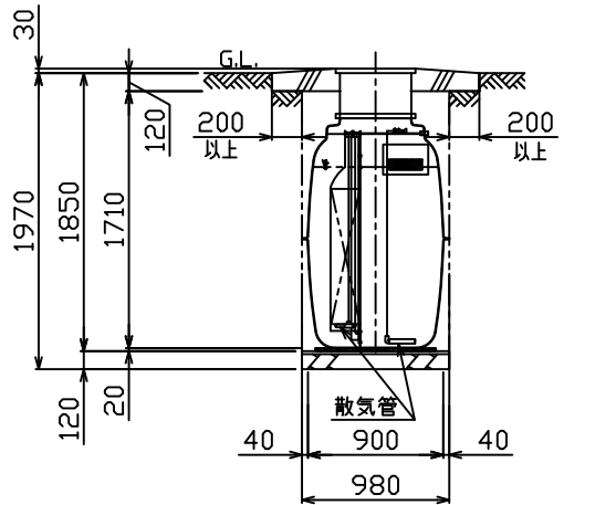
B - B断面図
