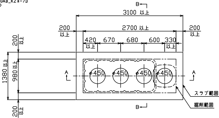
頂版開口図
